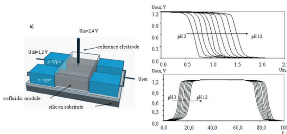
Рис. 1. рН-сенсора на основе комплементарной пары кремниевых ленточных полевых ионно-чувствительных транзисторов, где а) - внешний вид (эскиз) рН-сенсора, б) передаточная характеристика, в) временной отклик сенсора для треугольного входного импульса с амплитудой 2.4 В и длительностью 96 мс
