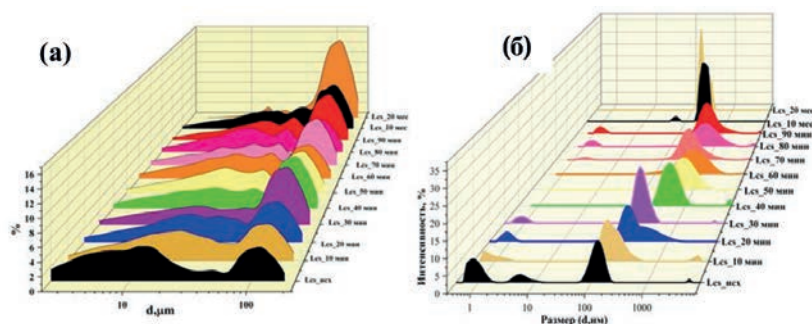
Рисунок. Эволюция дисперсных свойств водных растворов нагруженного лакосамида во времени по данным методов SLS (а) и DLS (б).
