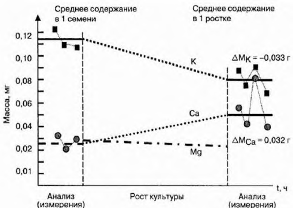
Рис. 2-1-2. Изменение содержания K, Ca, Mg при прорастании семян. Происходит реакция K39+p1=Ca40 .
