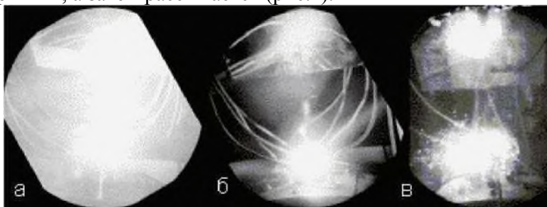
Рис. 1-7-2. "Странное" излучение, возникающее во время разрыва тока. На рисунке видно, что свечение возникает в центре между электродами над диэлектрической крышкой и имеет шарообразную форму.
