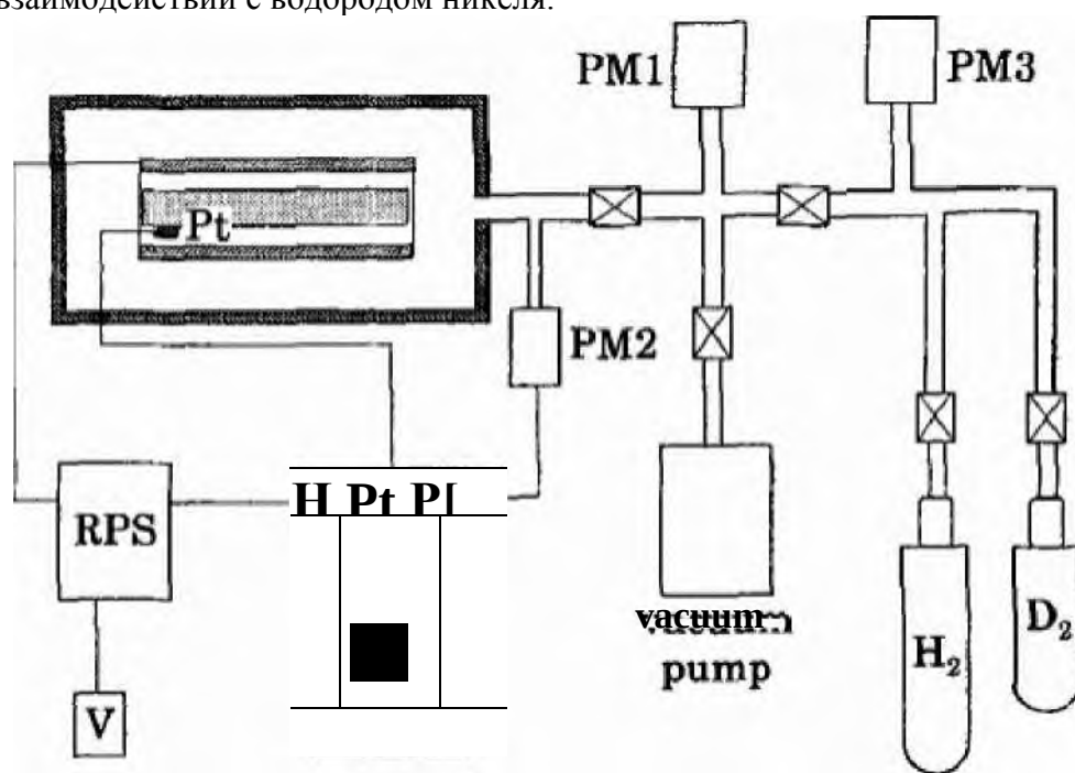
Рис. 1-4-5. Схема экспериментальной установки.
