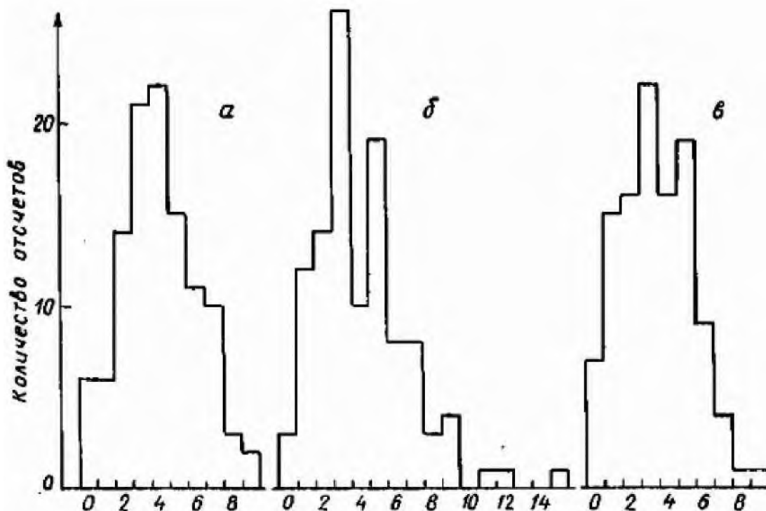
Рис. 3-2-1. Гистограмма фона (а), гистограмма воздействия (б), гистограмма последствия (в).
