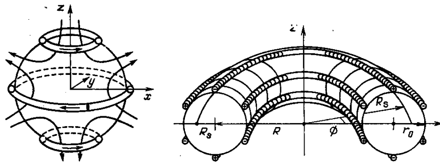
Рис. 14. а – секступольная сфера, б – секступольный тор
