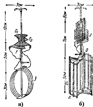
Рис. 25. а) магнитный резонатор, б) электрический резонатор
