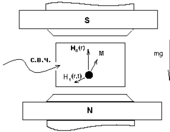
Рис.30. Схема опыта по левитации в условиях ф.м.р.
