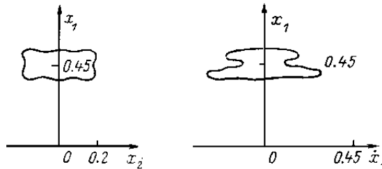
Рис. 33. Устойчивые траектории при \omega = 0.1\omega_1 , x_{10}'=-0,07 , x_{10}=0,2 , x_{20}'=-0,07 , x_{20}=0,11
