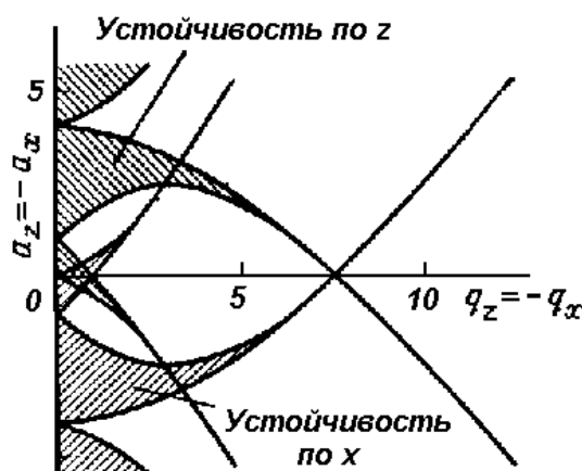
Рис.9. Полная диаграмма устойчивости для двухмерного квадрупольного поля
