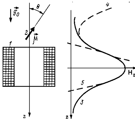
Рассмотренные примеры позволили предположить существование устойчивых состояний движений в зонах параметрического резонанса, что и было продемонстрировано в работе [84]. В качестве модели рассматривалось движение магнитного диполя в поле силы тяжести и переменном магнитном поле, создаваемом соленоидом.
