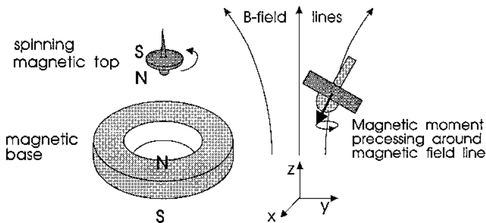
Рис. 17. Levitron
