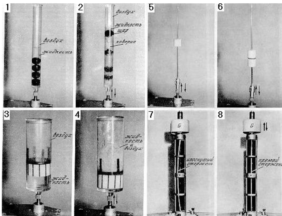
Рис. 6.1 – 6.8. «Маятники» Челомея
