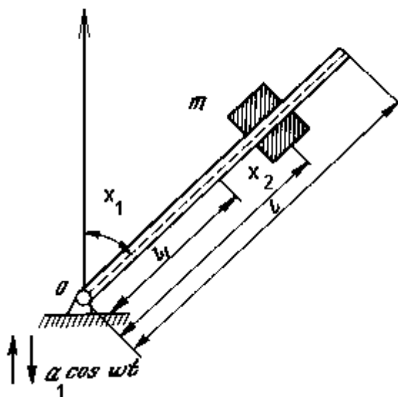
Рис.7. Маятник Челомея
