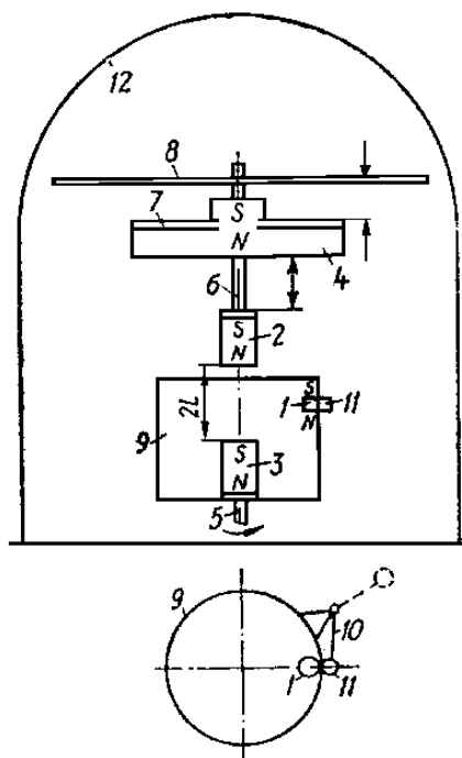
Рис.20. Опыт орбитального полета свободного магнита
