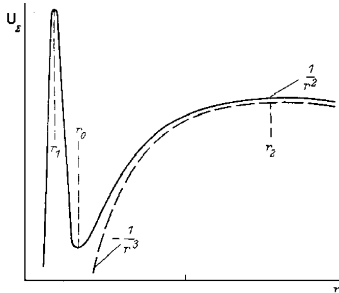
Рис. 31. Усредненная эффективная потенциальная энергия макроскопической спиновой частицы, находящейся в неоднородном магнитном поле ( \sim \mu_2 / r^3 ) и ВЧ-резонансном поле с \omega = \gamma \mu_2 / r^3
