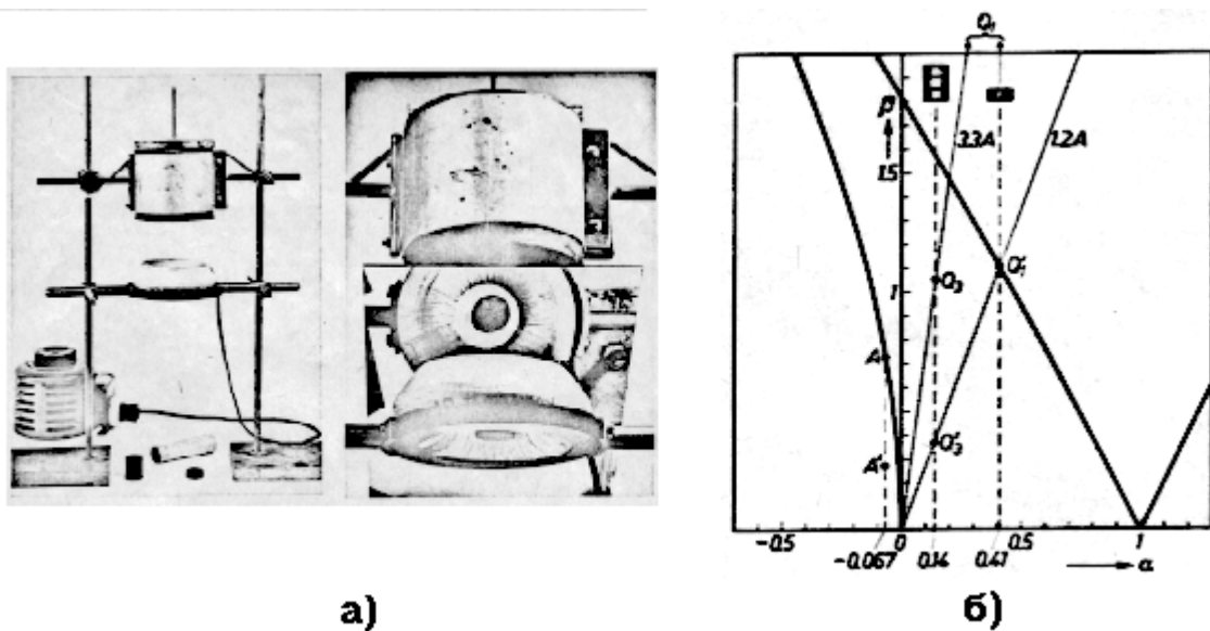
Рис. 15: а – магнитная ловушка [36], б – зоны устойчивого взвешивания
