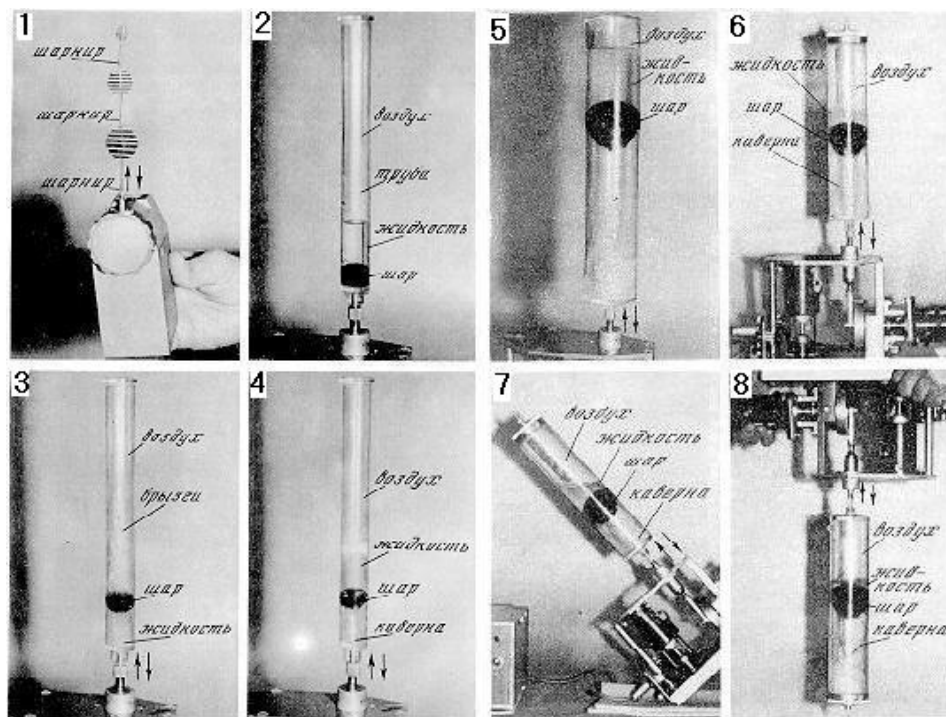
Рис. 5.1 – 5.8. «Маятники» Челомея
