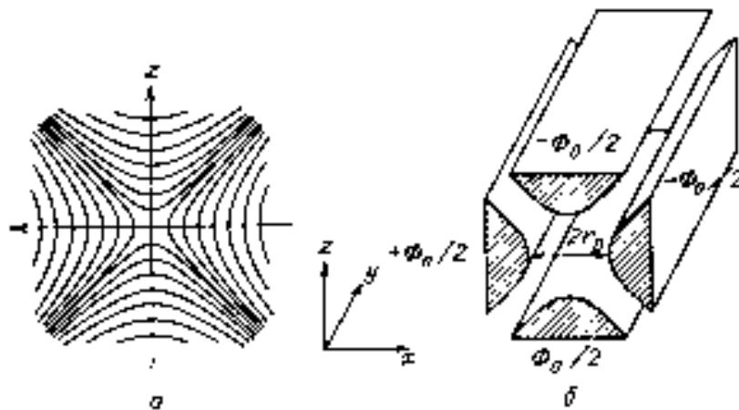
Рис. 8. Двумерный квадруполь
