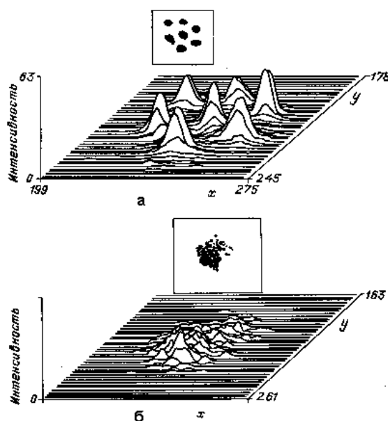
Рис. 12. а – псевдокристалл из семи ионов магния. Расстояние между частицами 23 мкм; б – те же частицы при более «высокой температуре». Кристалл расплавился
