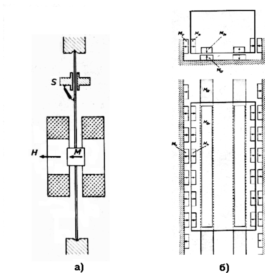
Рис. 16. Удержание движущегося постоянного магнита в поле неподвижного постоянного магнита (а – принцип, б –реализация)
