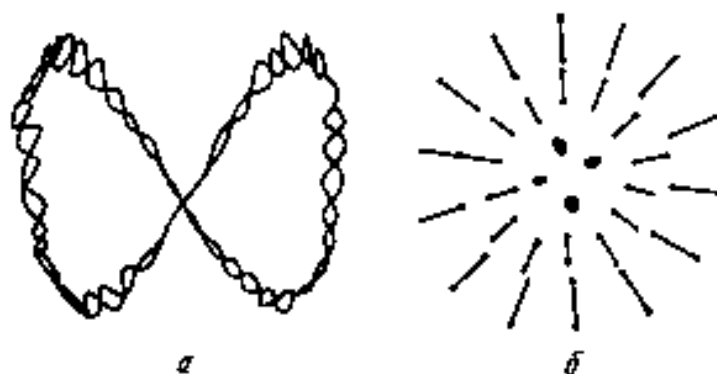
Рис.11. а – Микрофотография орбиты Лиссажу в плоскости r, z отдельной заряженной частицы порошка алюминия. Видно микродвижение. б – Картина "конденсированных" частиц алюминия
