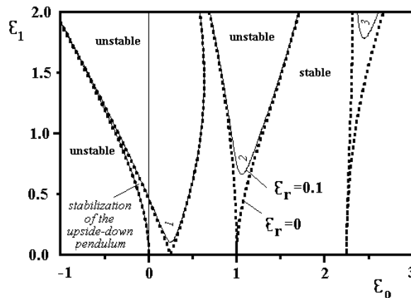
Рис. 2. Зоны параметрического резонанса
