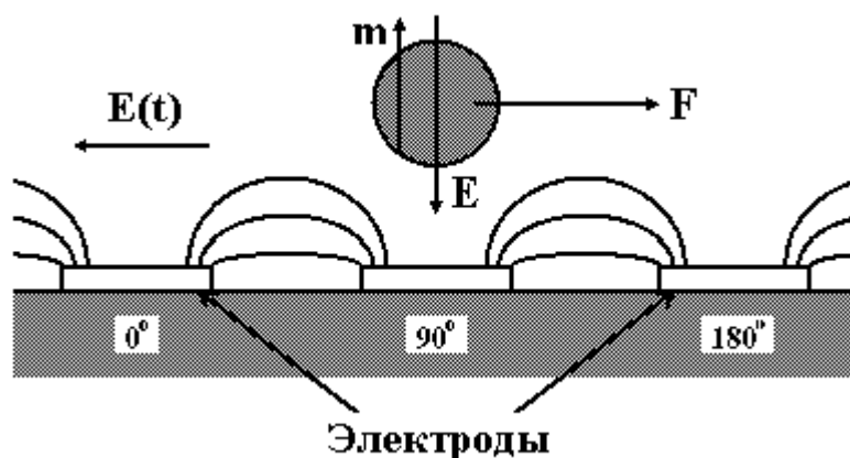
Рис. 23. Диэлектрфорез – «бегущая по волнам»
