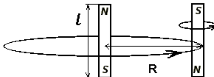
Рис. 19. Орбитальная устойчивость в системе из двух магнитов
