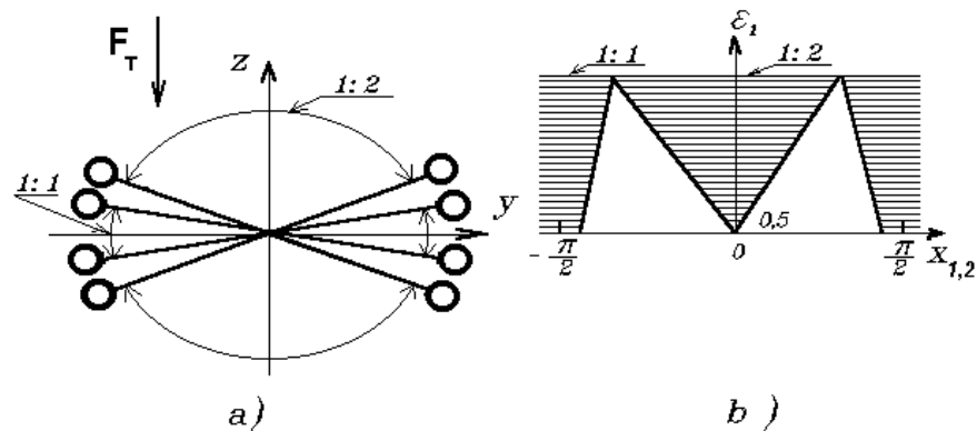
Рис. 29. Сценарий появления бифуркации для перевернутого маятника по Пуанкаре при \epsilon_0=0 . а) 0,5 < \epsilon_1 < 0,61 ; б) графики зависимости x_{1,2}(\epsilon_1)
