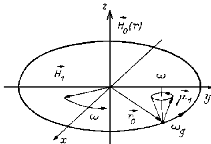
Рис. 32. Устойчивое движение в точке r_0 при резонансном захвате
