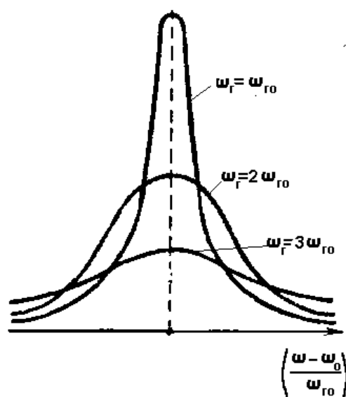
Рис. 27. Графики зависимости сил давления от расстройки по частоте при различных временах затухания 1/\omega_r
