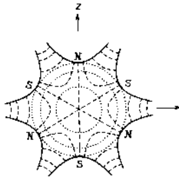
Рис. 13. Идеальное секступольное поле. Штриховые линии – линии магнитного поля, пунктир – линии равного магнитного потенциала, B = \text{const}
