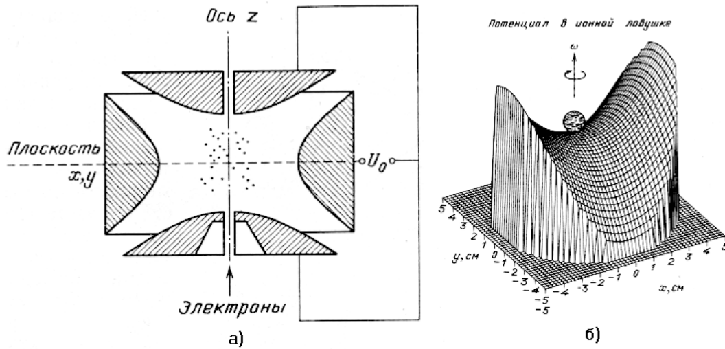
Рис.10. Ионная ловушка (а) и ее механический аналог (б)
